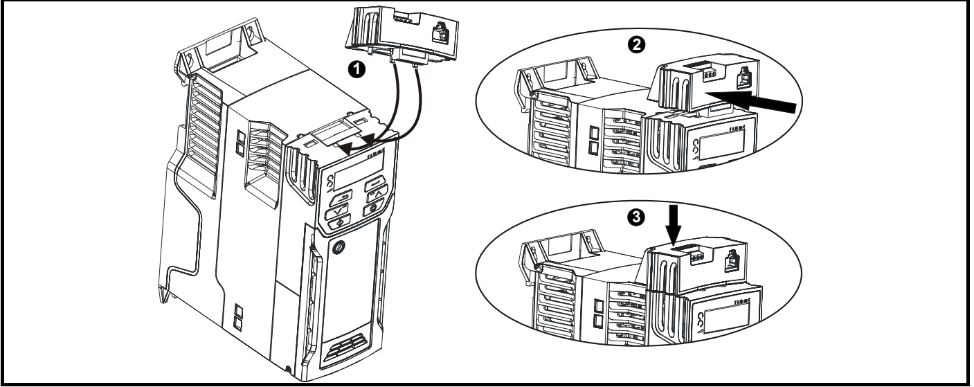
Şekil 3-5 AI-485 / AI-Backup Adaptörünü sürücüye yerleştirme (AI-485 Adaptörü gösterilmiştir)
